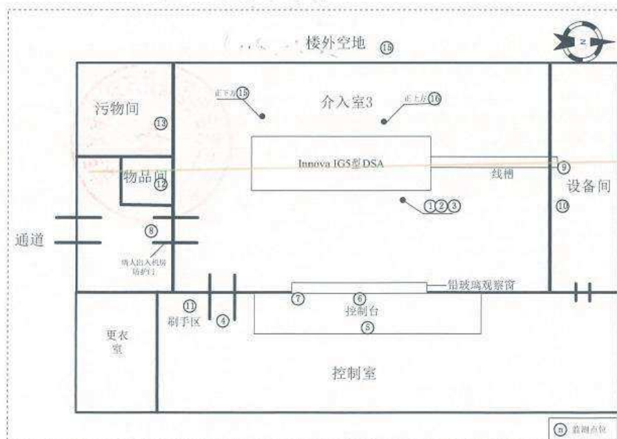
图 1 Innova IG5 型 DSA 应用场所监测点位布置图 (透视状态)
